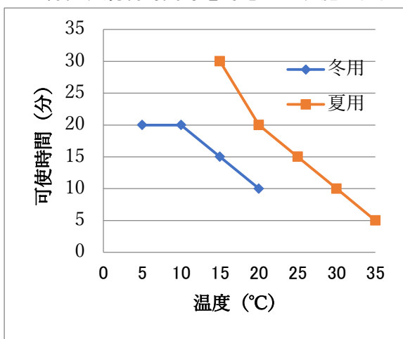
図-2 カラープライマ、バインダ樹脂の可使用時間
