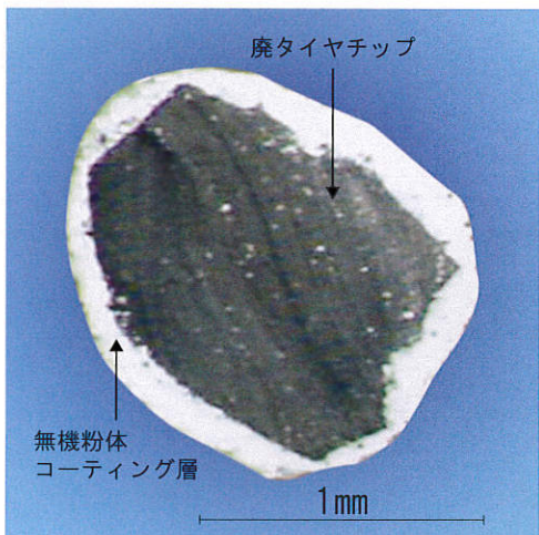
<PRMS弾性骨材 断面図>
